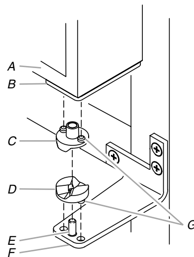
A. Châssis de porte B. Plaque de pivot C. Ferme-porte - partie supérieure D. Ferme-porte - partie inférieure E. Cheville de pivotement F. Charnière inférieure G. Pitons
