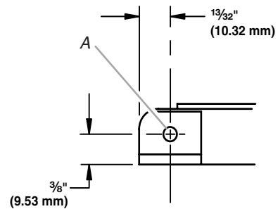
A. Top hinge-pin hole
