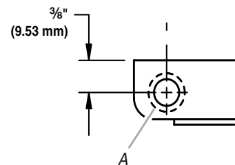
A. Bottom hinge-pin hole
